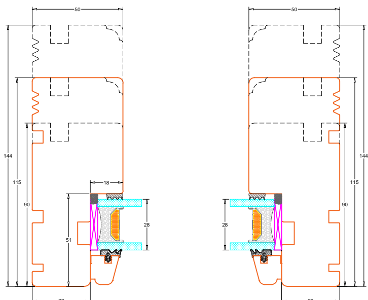
V1: Sidekarme faste partier
