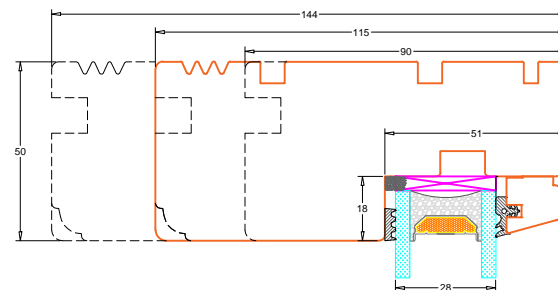
V2: Topkarm faste partier
