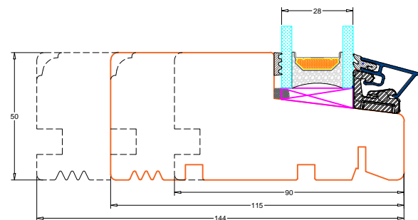
V5: Topkarm åbenbare eller faste partier med ramme
